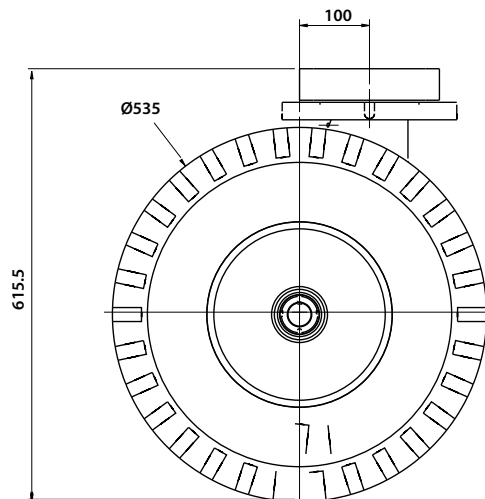
RAD-GESICHTSBREMSE OPTION - Zusatz, WFB'
